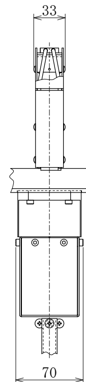
矢視 C
